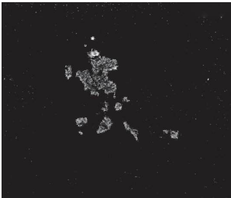
附图1b 用慢镜头拍摄下来的一个布朗粒子
