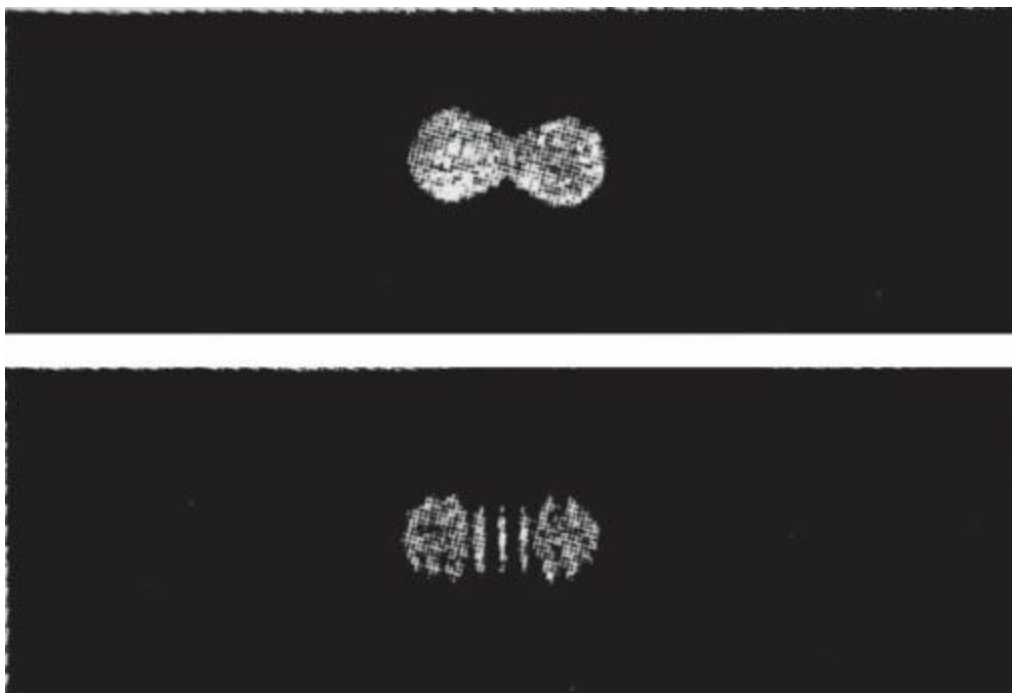
附图IIa 上面的照片是两束光通过两个紧挨着的小孔后所得到的光斑（先打开一个小孔，然后把它关上再打开另一个）。下面的照片是让光同时通过两个小孔所得到的光带 [ V. 阿尔卡迪耶 ( V. Arkadiev ) 摄 ]
