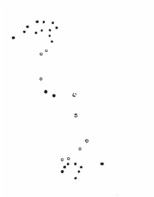
附图1c 从许多布朗粒子中认定一个粒子进行观察所得到的连续位置
