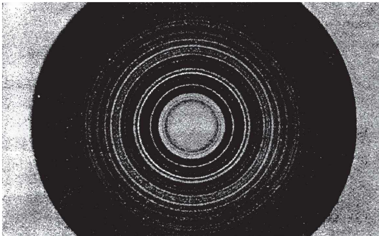
附图IIIc 电子波的衍射 [ 圣洛里亚及克林格 ( Klinger ) 摄 ]
