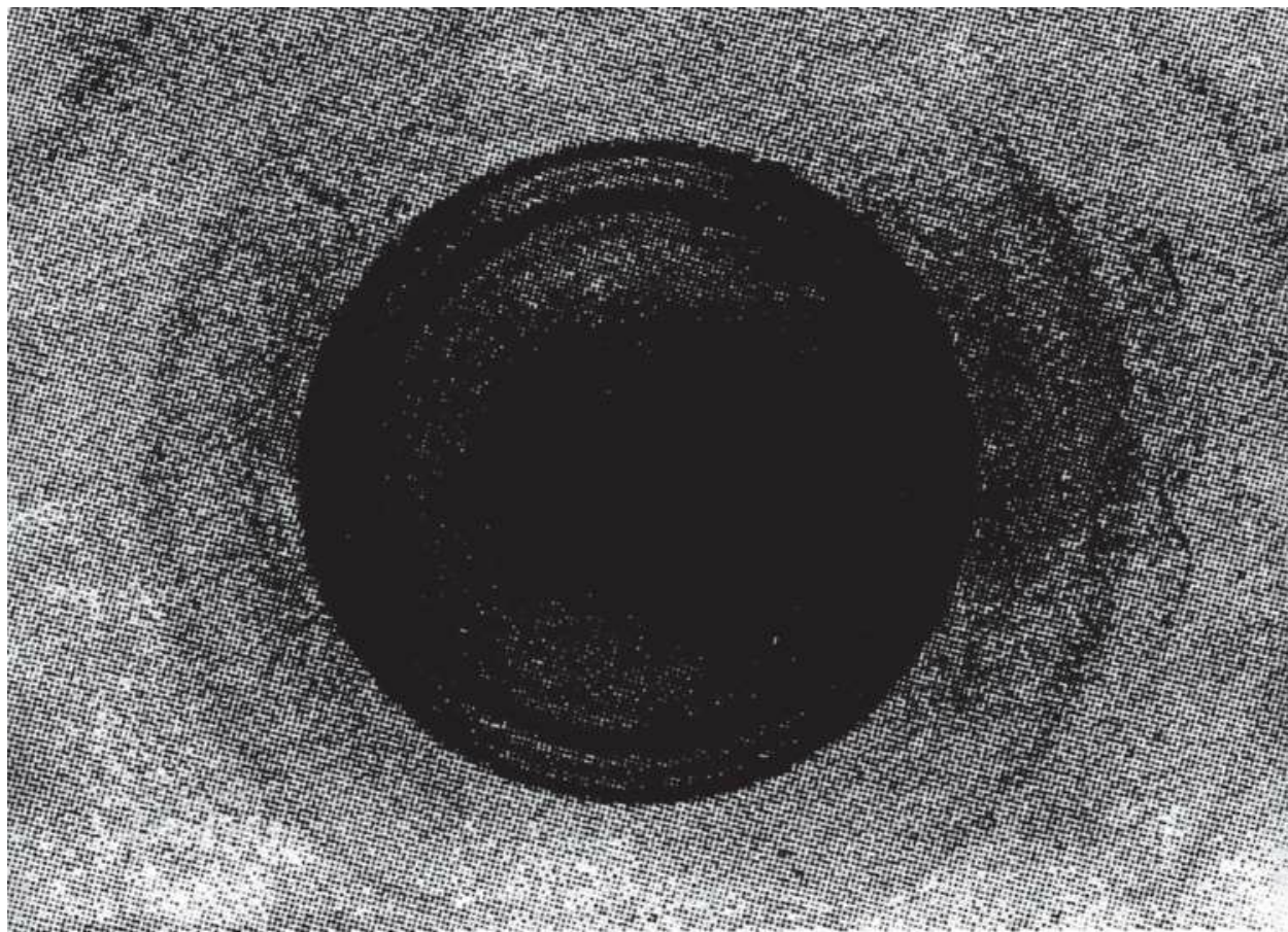
附图IIIb 射线的衍射 [ 拉斯托维金 ( Lastlowiecki ) 及格雷戈尔 ( Gregor ) 摄 ]
