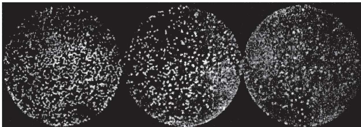
附图1a 显微镜中看到的布朗粒子 [ F.佩林 ( F. Perrin ) 摄 ]
