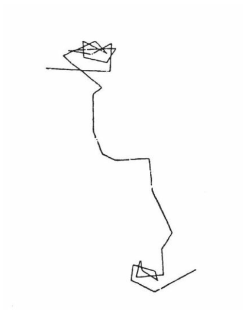
附图1d 从这些连续位置平均出来画成的路径
